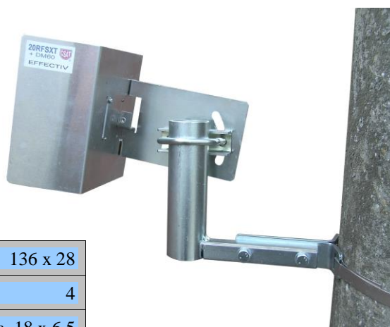
aplikácia KPRU60 TWIN montáž WiFi antény
