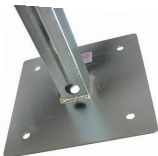
detail príruby konzoly NK
