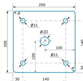
R = 5mm príruba NK montážne otvory majú priemer 11mm
