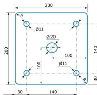
R = 5mm príruby NK montážne otvory majú priemer 11mm
