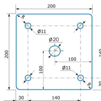
R = 5mm príruha KS7M-XP montážne otvory majú priemer 11mm
