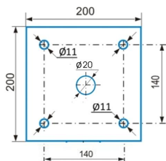
príruba KS3M-XP
