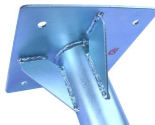
detail príruby
