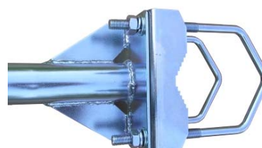
detail príruby s 2x Z5V105
