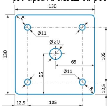
príruba KS-M
