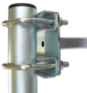
príruby KML300T + 2xVBZ3
