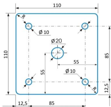
príruba KS
